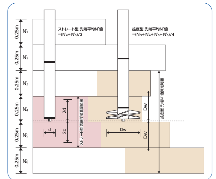
図1. 先端平均N'値の算定範囲
